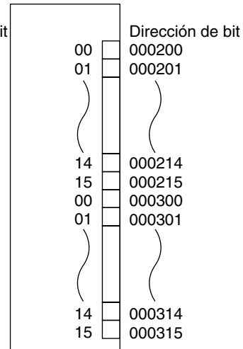
Posición 3 Unidad de entrada de c.c. de 32 puntos
