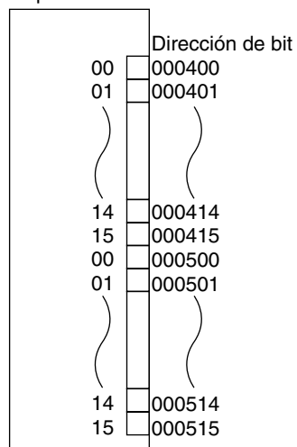
Posición 4 Unidad de salida transistor de 32 puntos
