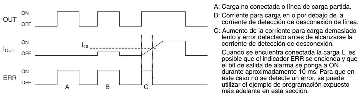
Figura 3: Desconexiones de línea
