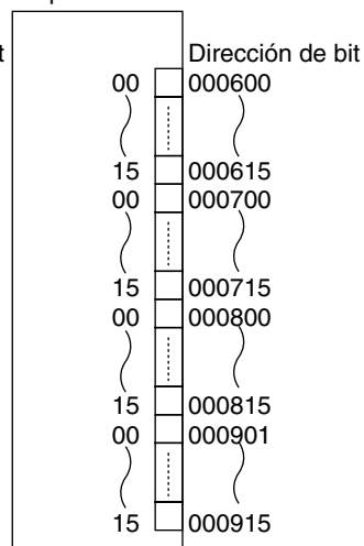
Posición 5 Unidad de salida transistor de 64 puntos
