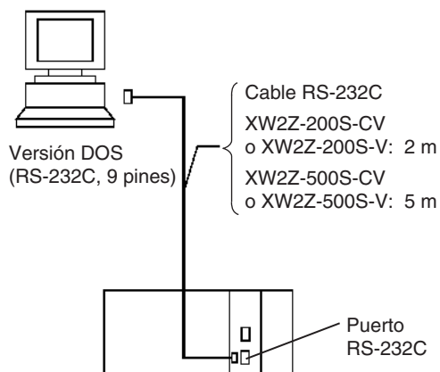
Cables de conexión del puerto RS-232C
